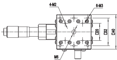
NFP-1461SL
