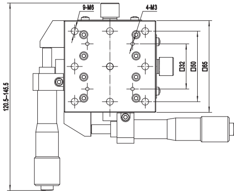
NFP-1462SL × 2
