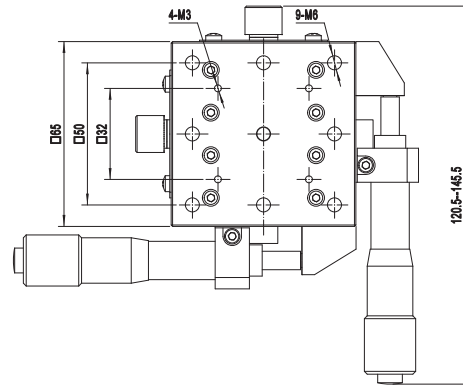
NFP-1462SR × 2
