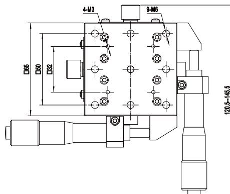
组维产品 NFP-1462SR直线滑台 × 2
